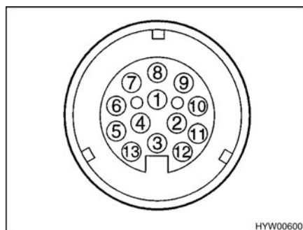
Fig. 108 Coupe de la prise du véhicule tracteur (système à 13 pôles de Jaeger)
