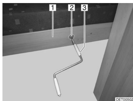
Fig. 72 Manivelle
