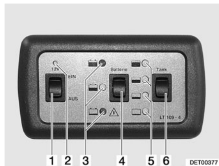
Fig. 99 Panneau de contrôle LT 109
