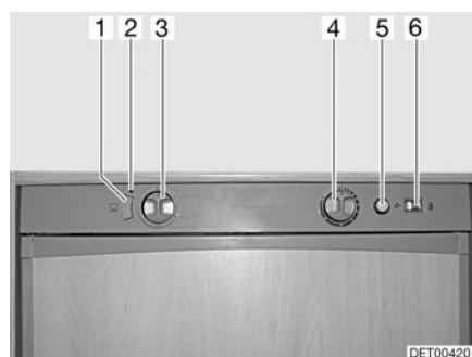
Fig. 146 Boutons de commande pour le réfrigérateur (Dometic série 7 avec allumage manuel et chauffage du cadre)
