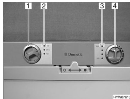
Fig. 147 Boutons de commande pour le réfrigérateur (Dometic Série 7 avec AES)
