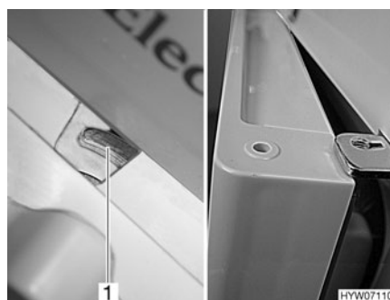
Fig. 186 Porte du réfrigérateur en position de ventilation (Dometic Série 7)
