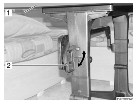
Fig. 76 Dispositif de verrouillage table pivotante sans étrier
