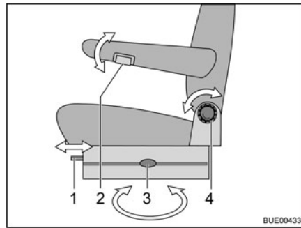
Fig. 8 Siège conducteur et siège passager (Aguti)
