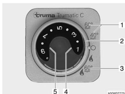
Fig. 169 Unité de commande pour chauffage/chauffe-eau
