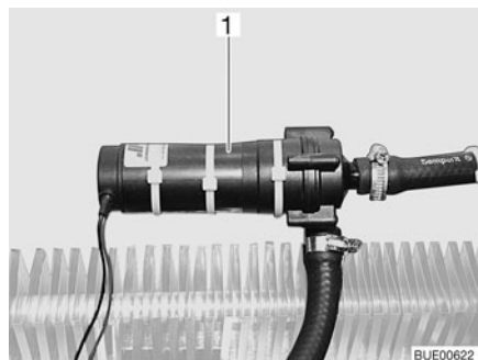
Fig. 155 Circulateur supplémentaire
