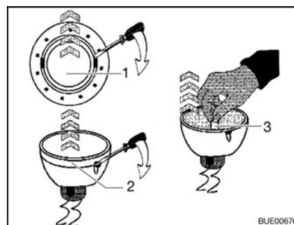
Fig. 235 Remplacer l'ampoule halogène
