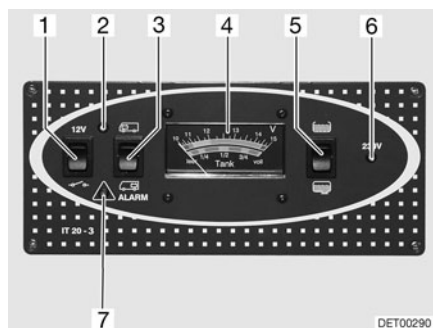
Fig. 129 Panneau de contrôle IT 20-3
