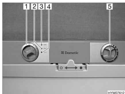
Fig. 182 Boutons de commande pour le réfrigérateur (Dometic Série 7)
