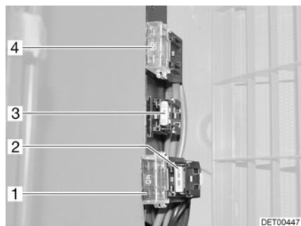
Fig. 139 Fusibles de la batterie de cellule (Fiat)
