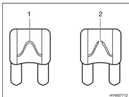
Fig. 135 Fusible 12 V
