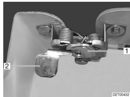
Fig. 21 Bouton de déverrouillage extérieur du capot moteur
