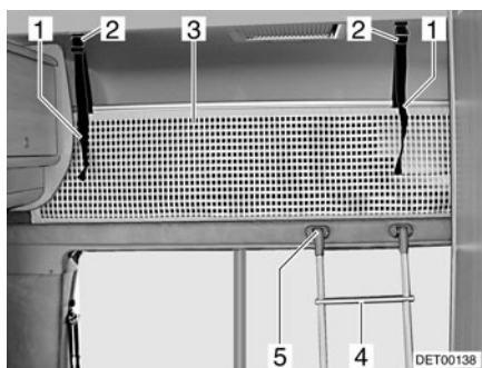
Fig. 88 Lit de capucine
