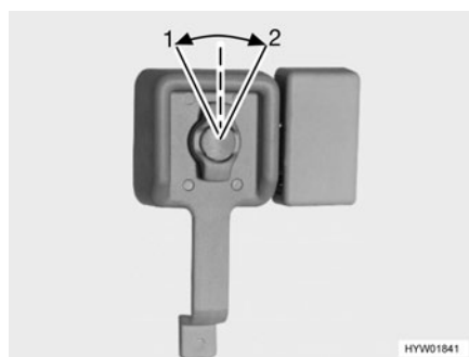
Fig. 31 Serrure de la porte cellule, à l'intérieur, ouverte
