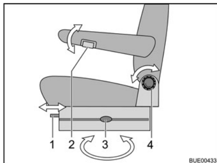
Fig. 68 Siège conducteur et siège passager (Aguti)
