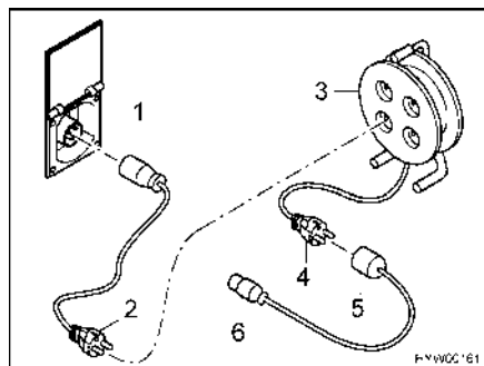
Fig. 133 Possibilités de raccordement 230 V
