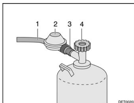
Fig. 122 Raccord bouteille de gaz
