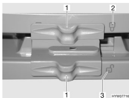
Fig. 187 Verrouillage de la porte du réfrigérateur/du compartiment congélation (Dometic Série 7 avec compartiment congélation séparé)
