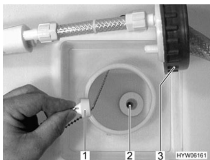
Fig. 196 Bouchon de fermeture
