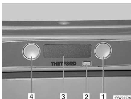
Fig. 184 Boutons de commande pour le réfrigérateur (Thetford sans SES)
