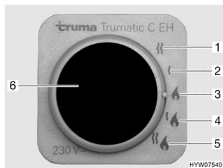
Fig. 171 Sélectionneur de source d'énergie pour chauffage/chauffe-eau
