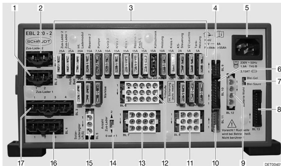
Fig. 128 Bloc électrique (EBL 220)
