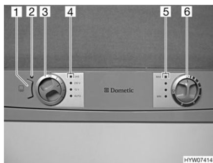
Fig. 183 Boutons de commande pour le réfrigérateur (Dometic Série 7 avec AES et CC)
