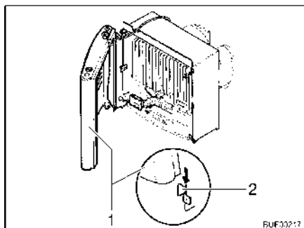
Fig. 115 Habillage du chauffage, pattes de retenue
