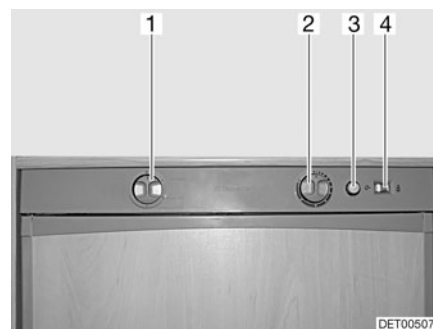
Fig. 145 Boutons de commande pour le réfrigérateur (Dometic Série 7 avec allumage manuel)
