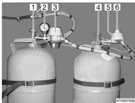
Fig. 93 Dispositif de commutation Duomatic
