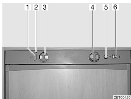
Fig. 146 Boutons de commande pour le réfrigérateur (Dometic série 7 avec allumage manuel et chauffage du cadre)
