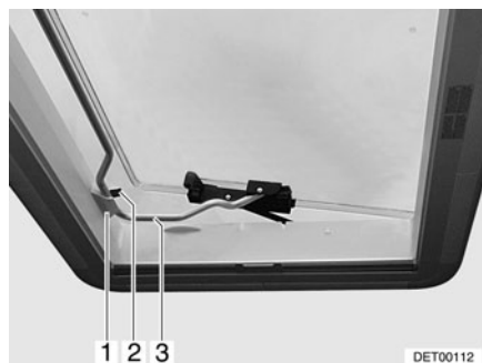
Fig. 55 Lanterneau Heki en position de ventilation 2
