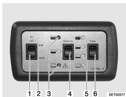
Fig. 99 Panneau de contrôle LT 109
