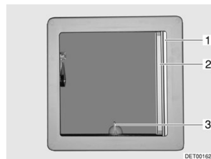
Fig. 48 Lanterneau basculant
