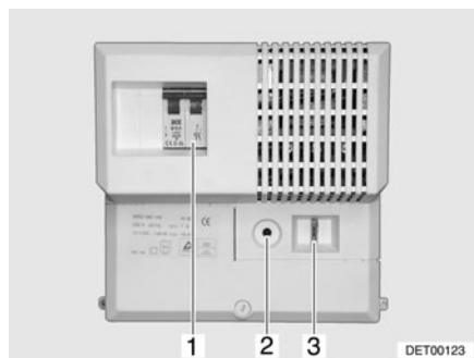
Fig. 95 Bloc transformateur
