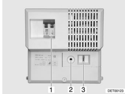
Fig. 106 Disjoncteur de protection de circuit (variante 1)
