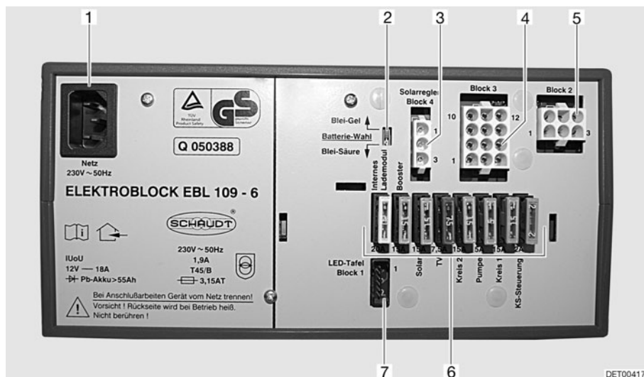
Fig. 98 Bloc électrique EBL 109
