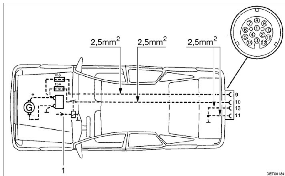
Fig. 109 Installation du véhicule tracteur (Pack Autarcie)
