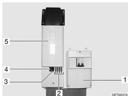
Fig. 96 Bloc transformateur (type I)
