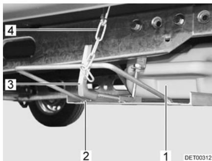
Fig. 159 Réservoir d'eaux usées dans le support sous le véhicule
