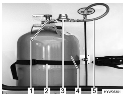
Fig. 90 Compartiment à gaz
