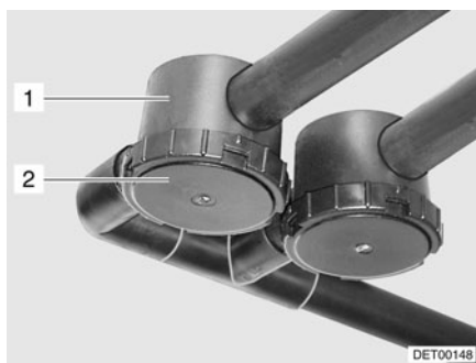
Fig. 160 Siphon
