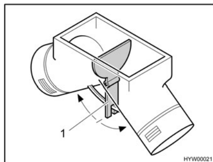
Fig. 119 Ventilateur à air pulsé, vanne de réglage en position intermédiaire
