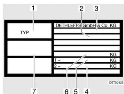
Fig. 191 Plaque signalétique
