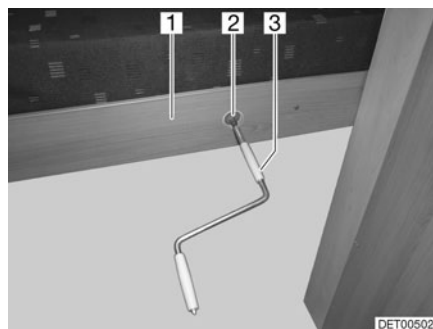
Fig. 72 Manivelle
