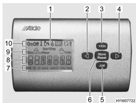
Fig. 121 Unité de commande pour le chauffage à eau chaude
