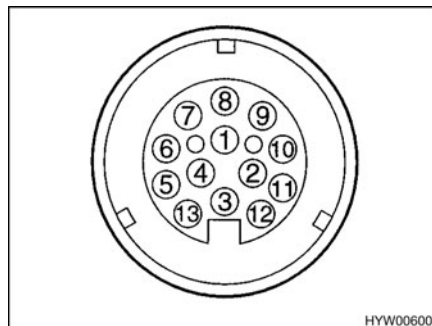
Fig. 108 Coupe de la prise du véhicule tracteur (système à 13 pôles de Jaeger)
