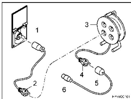
Fig. 101 Possibilités de raccordement 230 V
