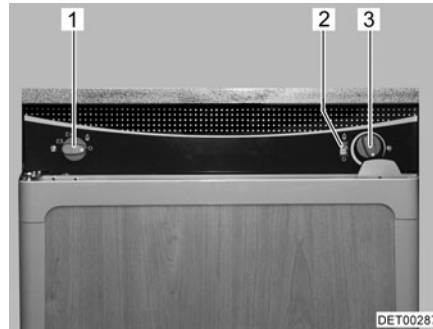
Fig. 148 Boutons de commande pour le réfrigérateur (Thetford sans SES)
