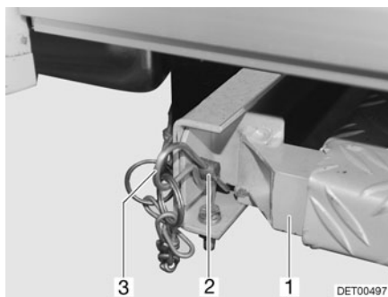
Fig. 6 Verrouiller la rampe mobile
