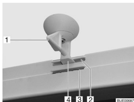
Fig. 47 Lanterneau basculant, dispositif de verrouillage
