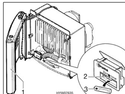
Fig. 114 Chauffage ouvert
