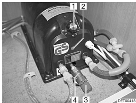
Fig. 133 Chauffe-eau Reich
