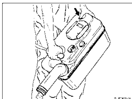
Fig. 171 Vidanger la cassette Thetford
