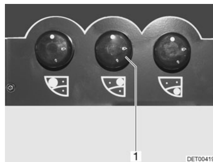
Fig. 137 Alternative : Boutons de commande pour le réchaud à gaz
