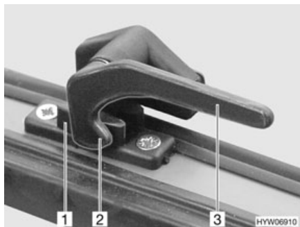
Fig. 51 Levier de verrouillage en position "Fermé"
