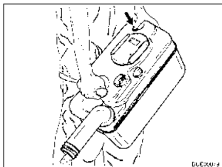
Fig. 263 Vidanger la cassette Thetford
