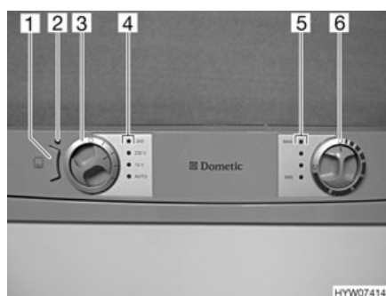
Fig. 212 Boutons de commande pour le réfrigérateur (Dometic Série 7 avec AES et CC)
