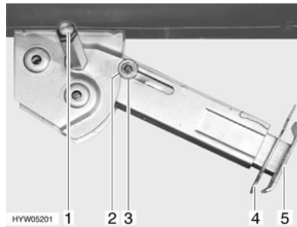
Fig. 32 Vérin stabilisateur
