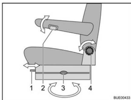
Fig. 73 Siège conducteur et siège passager (Aguti)
