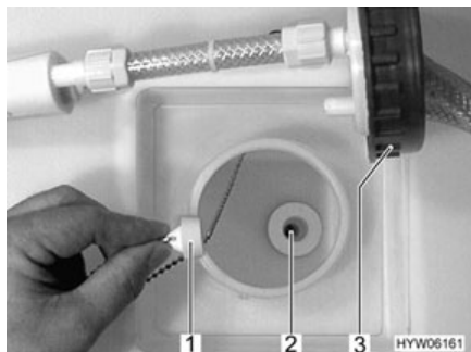
Fig. 232 Bouchon de fermeture
