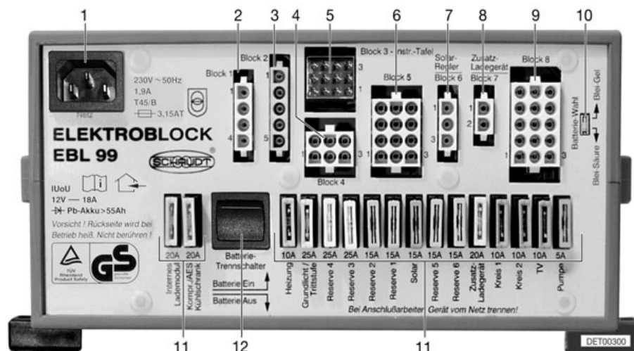
Fig. 157 Bloc électrique (EBL 99)
