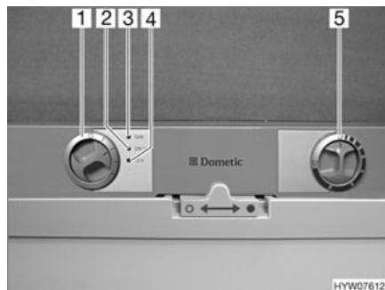
Fig. 211 Boutons de commande pour le réfrigérateur (Dometic Série 7)
