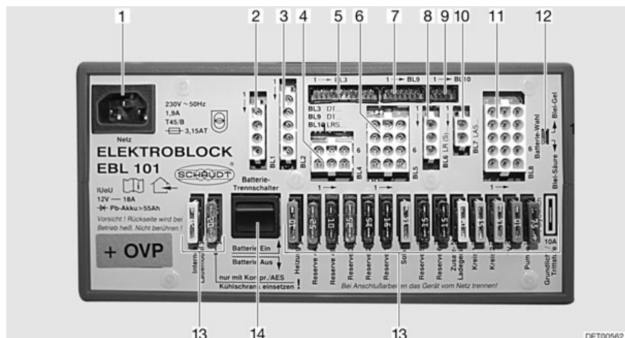
Fig. 158 Bloc électrique (EBL 101)
