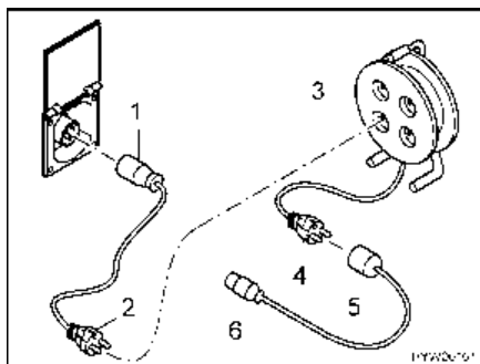
Fig. 162 Possibilités de raccordement 230 V
