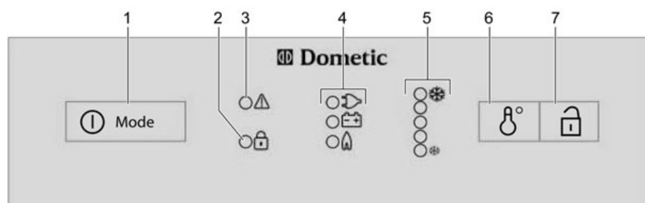
Fig. 214 Boutons de commande pour le réfrigérateur (Dometic Série 8 avec SMSE)
