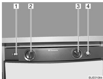
Fig. 213 Boutons de commande pour le réfrigérateur (Dometic Série 8)
