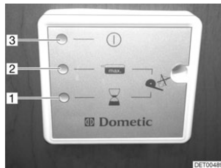
Fig. 258 Panneau toilette à aspiration
