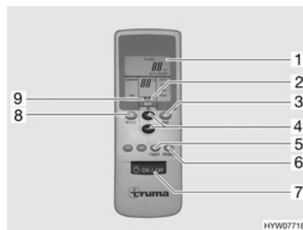
Fig. 194 Télécommande
