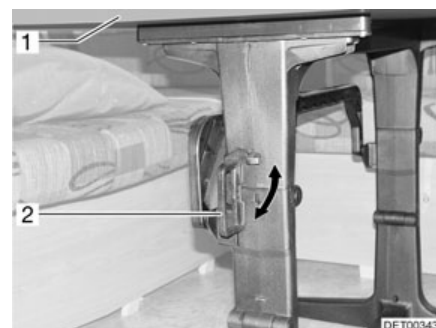
Fig. 84 Dispositif de verrouillage table pivotante sans étrier
