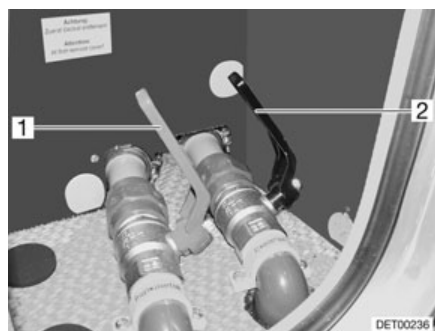
Fig. 235 Robinet d'évacuation des eaux usées
