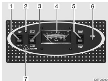
Fig. 159 Panneau de contrôle IT 20-3
